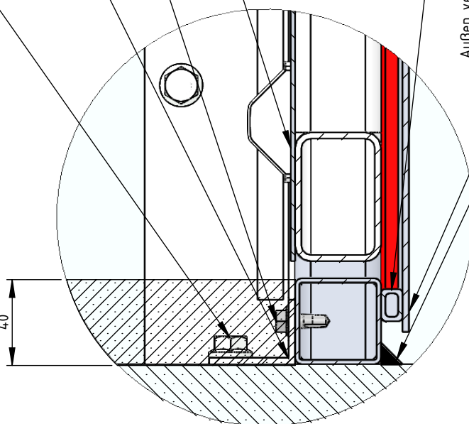
DETAIL E MAßSTAB 1 : 2.5
