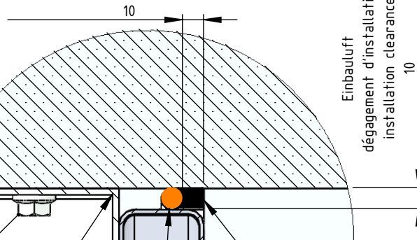
DETAIL F MAßSTAB 1 : 2.5
