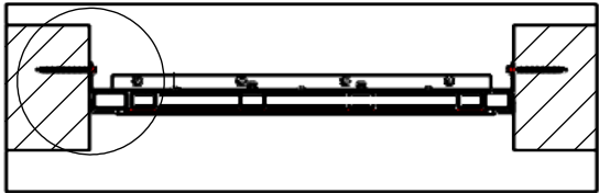
SCHNITT K-K
